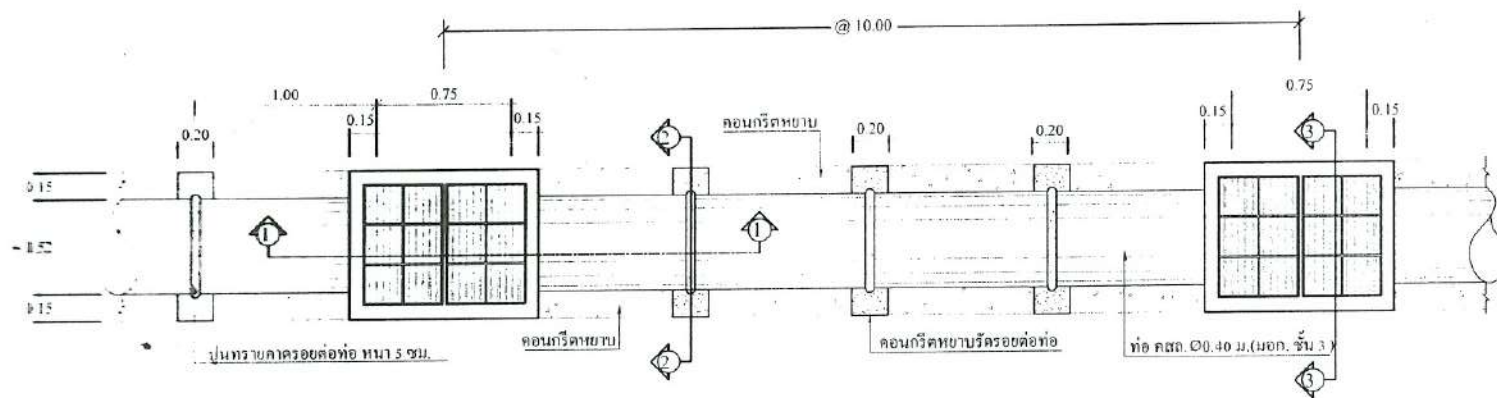
แปลนขยายวางท่อและบ่อพัก 1:20
