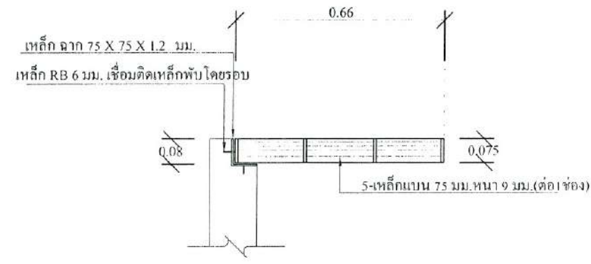
แบบขยายฝาบ่อพัก
