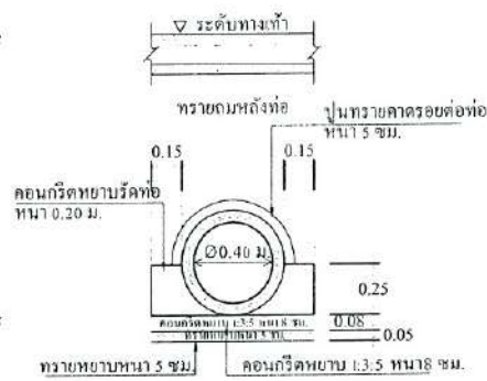
รูปตัดบ่อพัก 2-2 1:20
