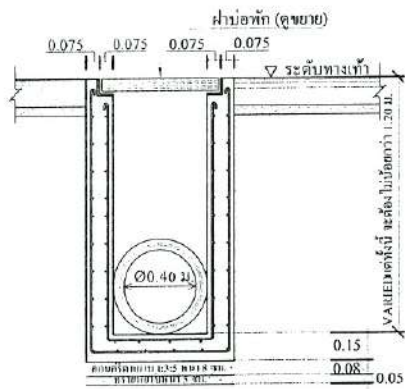
รูปตัดบ่อพัก 3-3 1:20
